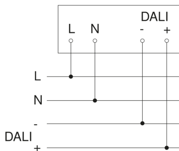
Schema elettrico Master
